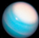
Uranus
